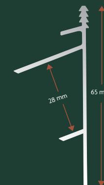
TILSLUTNINGSPROFIL NR 5307: For 28 mm tre
